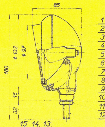
ROZMĚROVÝ NÁČRTEK – rozměry v mm:
